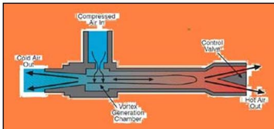
Fig. 1: Vortex Tube Schematic
